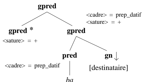
FIG. 4 – Arbre auxiliaire pour exprimer les compléments d'attribution.
